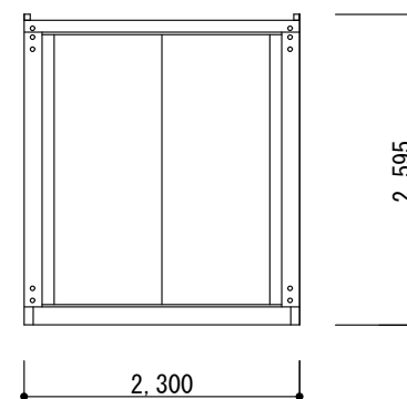
D 面 立 面 図
