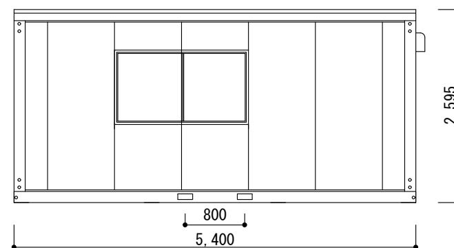
C 面 立 面 図
