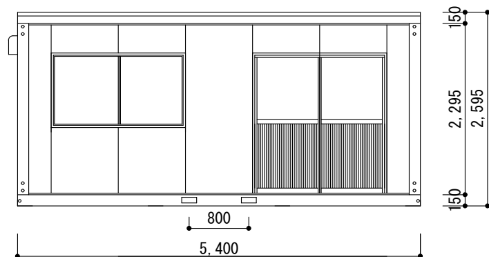
A 面 立 面 図
