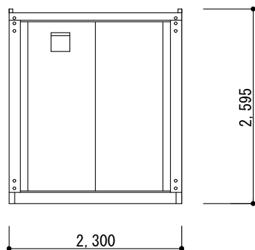
B 面 立 面 図
