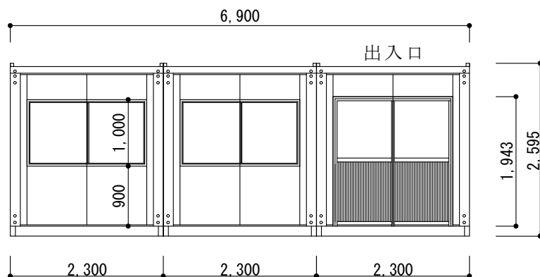
A 面 立 面 図
