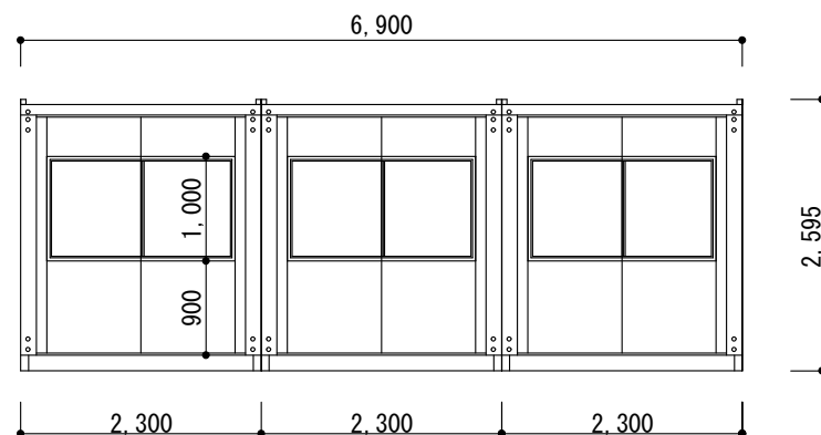
C 面 立 面 図
