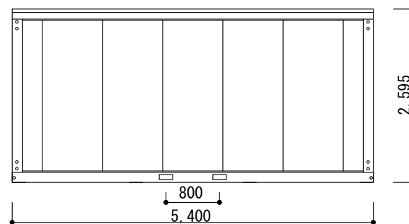
D 面 立 面 図
