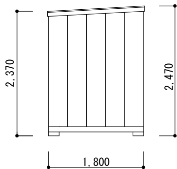
右側 立面図
