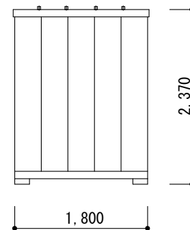
背面 立面図
