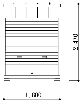
正面 立面図
