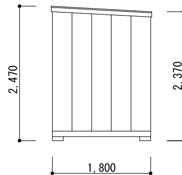
左側 立面図
