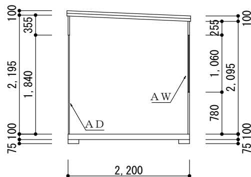
断 面 立 面 図
