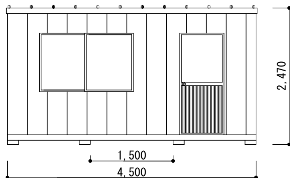
A 面 立 面 図
