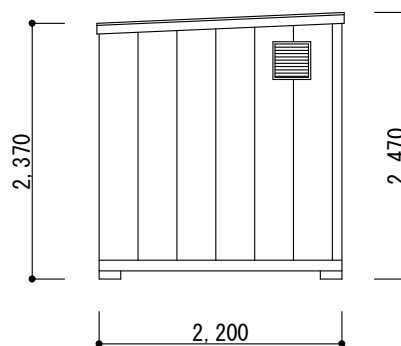
B 面 立 面 図
