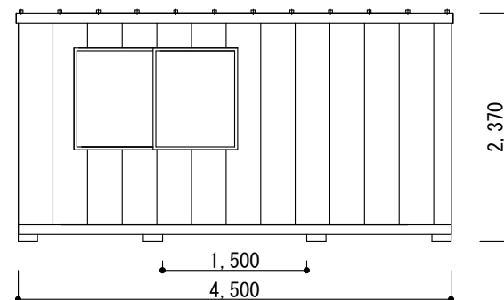
C 面 立 面 図
