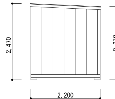
D 面 立 面 図
